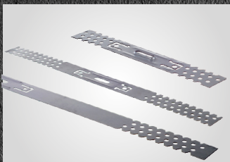
Wieszak ES ES hanger / ES Kleiderbügel
